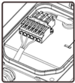
Réglage puissance 50% 75% 100%
